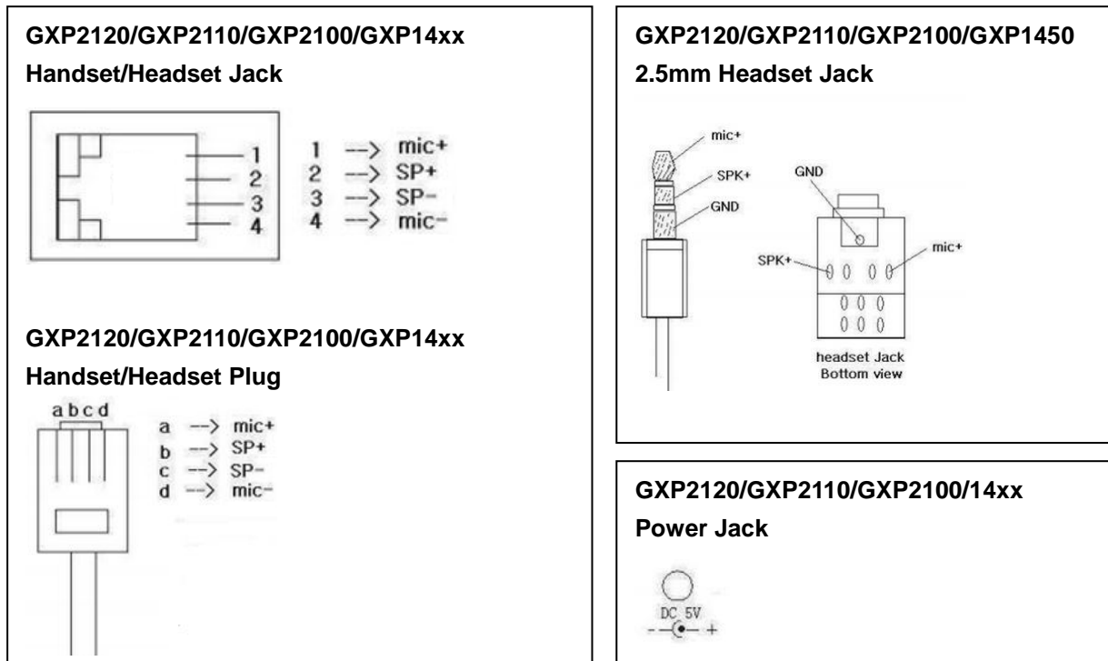
Figure 1: GXP2120/GXP2110/GXP2100/GXP14xx Pin-out
